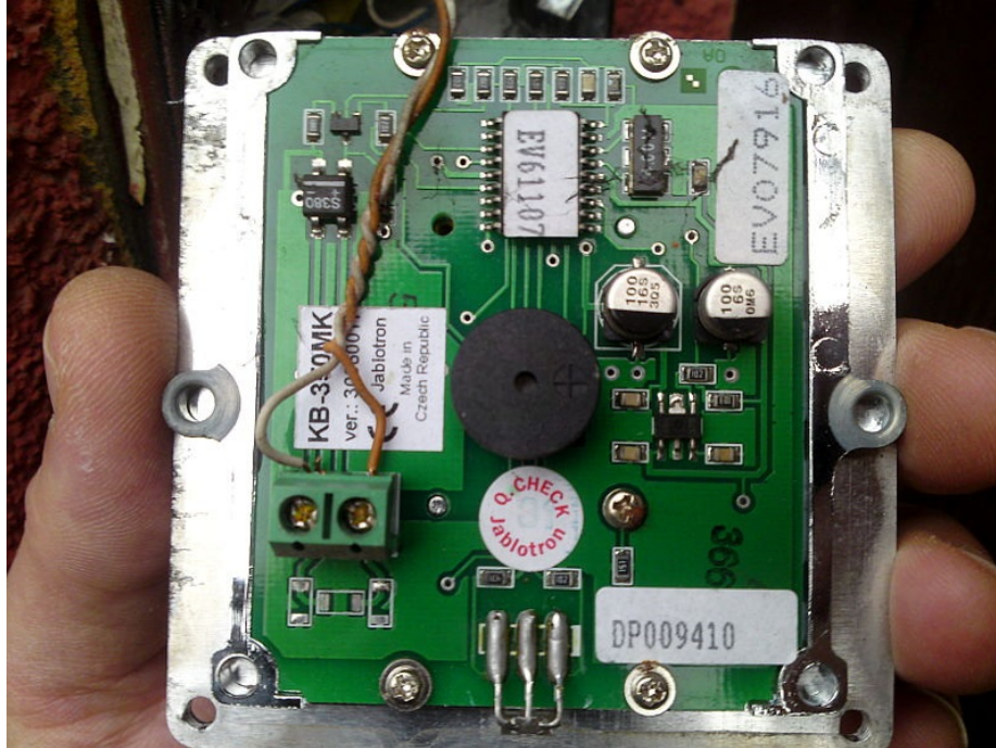
ovládací klávesnice
